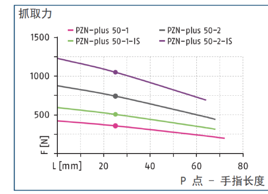
抓取力, 内撑抓取
